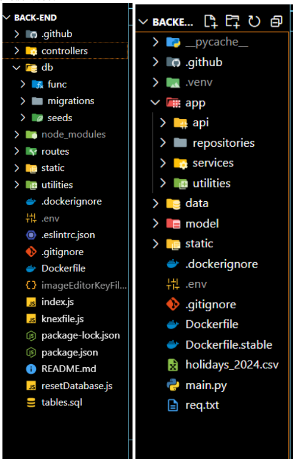
Gambar 6 hasil kode dari backend
