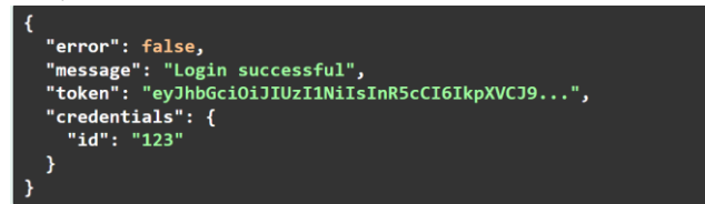
Gambar 8 contoh JSON hasil API.
