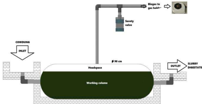
Gambar 1. 4. 1 Sistem Produksi Biogas Tetap
