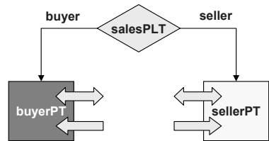
(b) scenario
