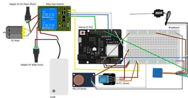
Gambar 3. 3 Perancangan Prototype
