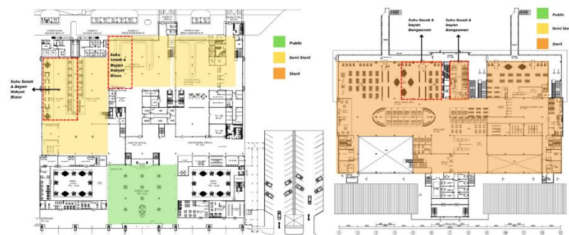
Gambar 1 Konsep organisasi ruang Lt. 1 & 2
