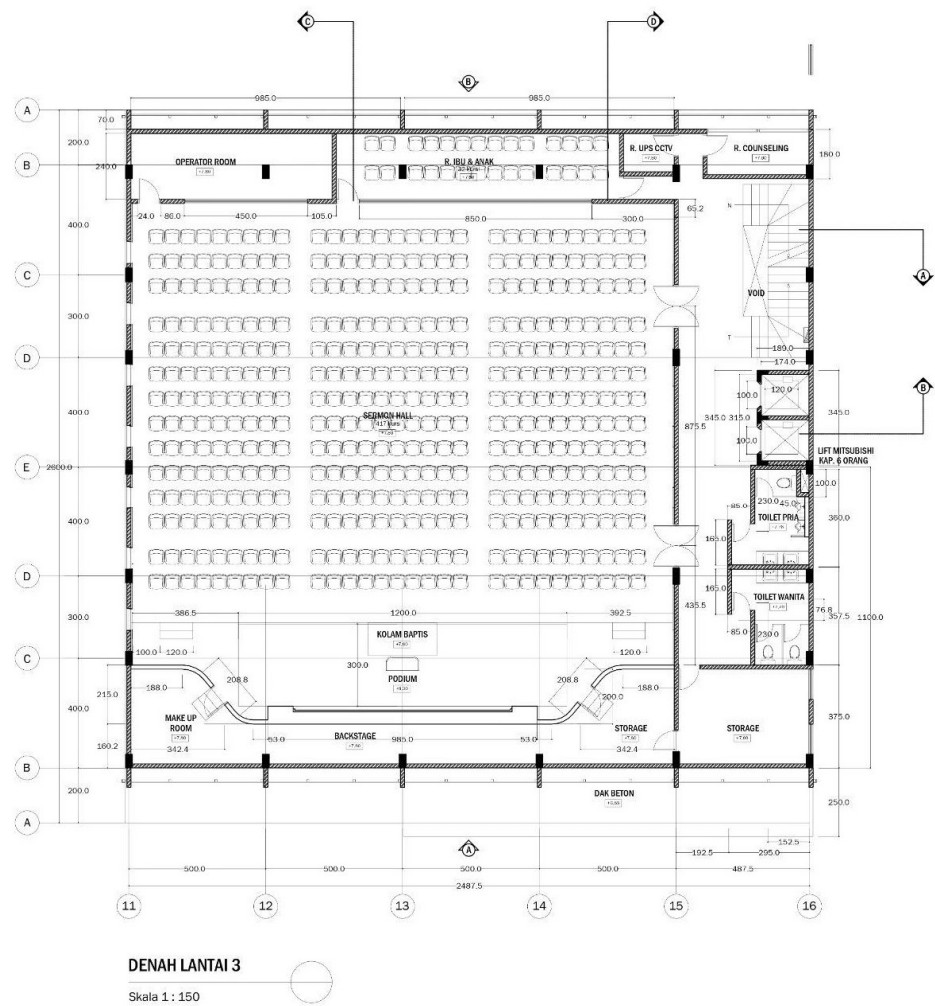
Gambar 1. 3 Denah Arsitek Lantai 3
