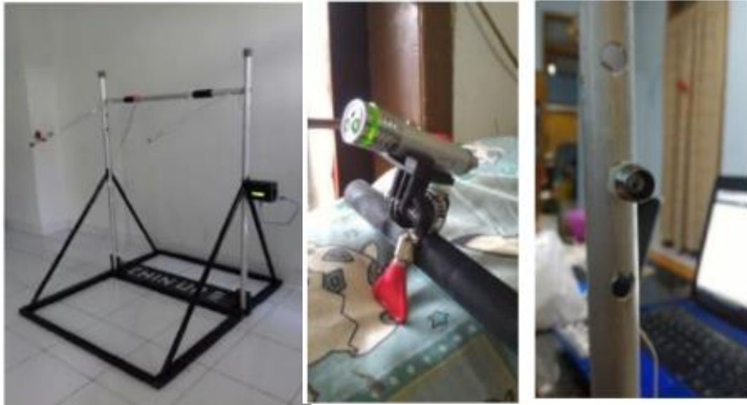
Gambar 1.2 Tes Chin-up Berbasis Arduino Uno dan Sensor Laser Infrared
