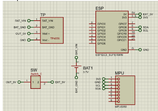
GAMBAR 1. Rangkaian Schematic
