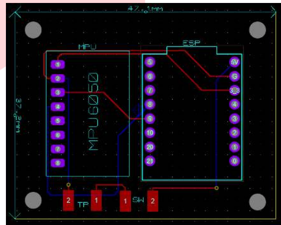
GAMBAR 2. Desain PCB
