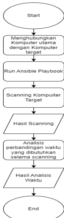
GAMBAR IV. 3 Flow Chart Pengujian Otomasi Ansible
