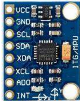
Gambar 2 2 Sensor MPU6050
