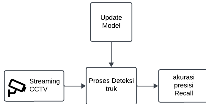
Gambar 7. Proses klasifikasi truk berbasis YOLOv8
