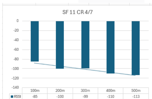
GAMBAR 18 (Grafik RSSI SF 11 CR 4/7)
