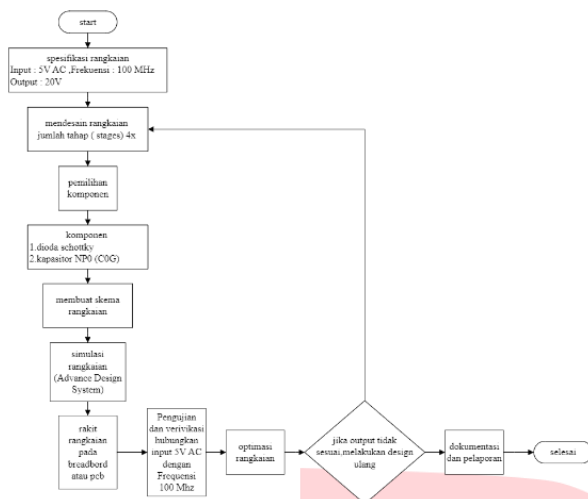
GAMBAR 7 (FLOWCHART Pengerjaan)
