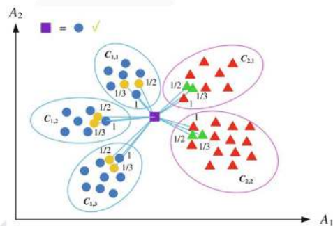
GAMBAR 2 Cara Kerja MVMCNN pada k=3
