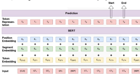
GAMBAR 1 Arsitektur BERT untuk sistem QA
