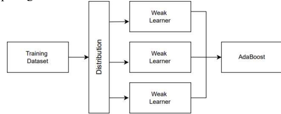
GAMBAR 2.2 Ilustrasi AdaBoost
