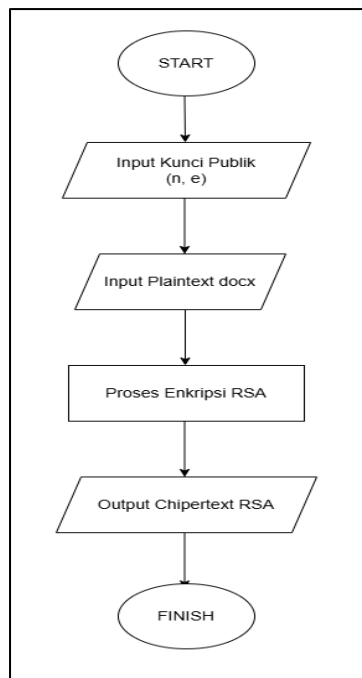
GAMBAR 4 (SKEMA ENKRIPSI RSA)
