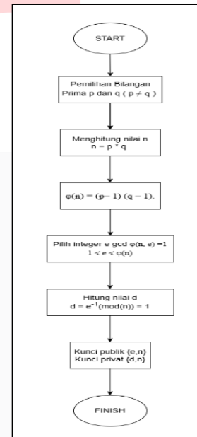
Gambar 3 (Skema Pembangkitan Kunci RSA)
