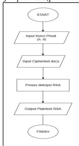
GAMBAR 5 (SKEMA DEKRIPSI RSA)
