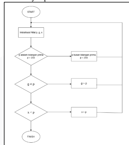
GAMBAR 6 (SKEMA PEMBANGKITAN KUNCI EL-GAMAL)
