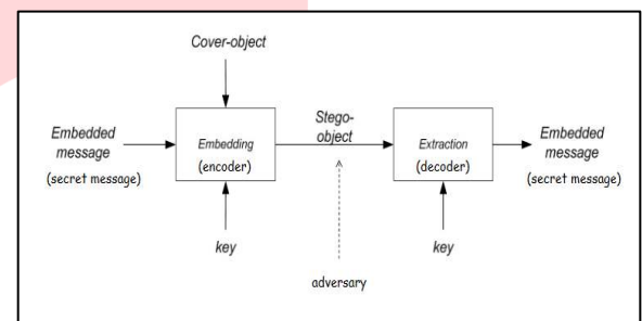
GAMBAR 9 (SKEMA STEGANOGRAFI)
