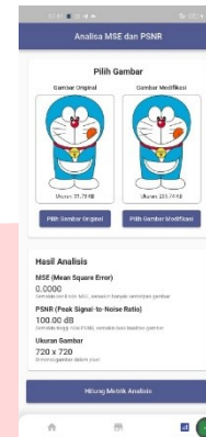
GAMBAR 7. (HASIL PENGUJIAN MSE DAN PSNR)
