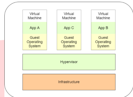
GAMBAR 2 (Skema Virtual Machine[12])
