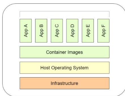
GAMBAR 1 (Skema Container[12])
