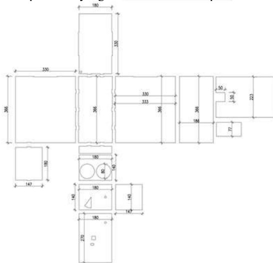
GAMBAR 2.1 Pola design sistem alat
