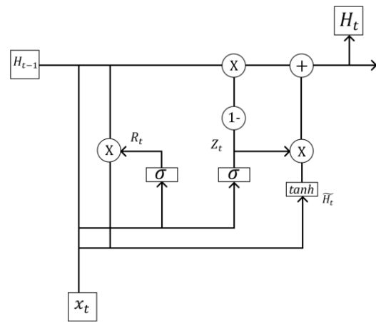
Fig. 1. Structure of GRU
