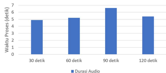
GAMBAR 7 Perbandingan Waktu Pemrosesan Terhadap Durasi Audio
