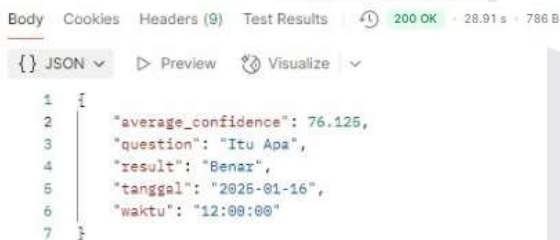
GAMBAR 5 Hasil Proses dari Postman Kondisi Server Sleep
