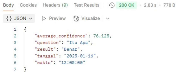
GAMBAR 3 Hasil Proses Dari Postman Kondisi Server Tidak Sleep
