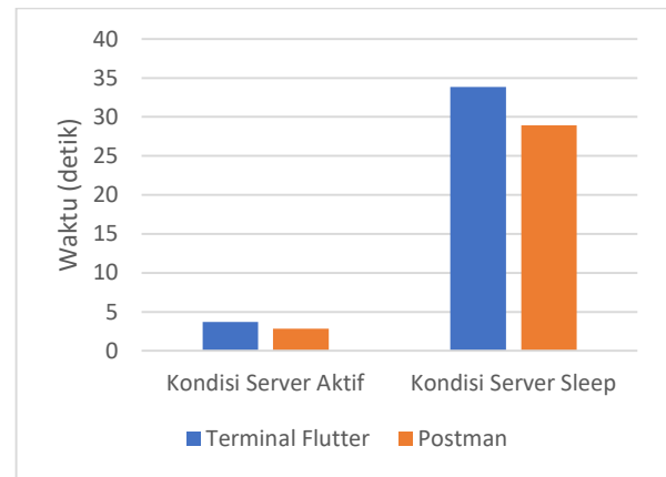
GAMBAR 6 Perbandingan Latensi Terhadap Kondisi Server
