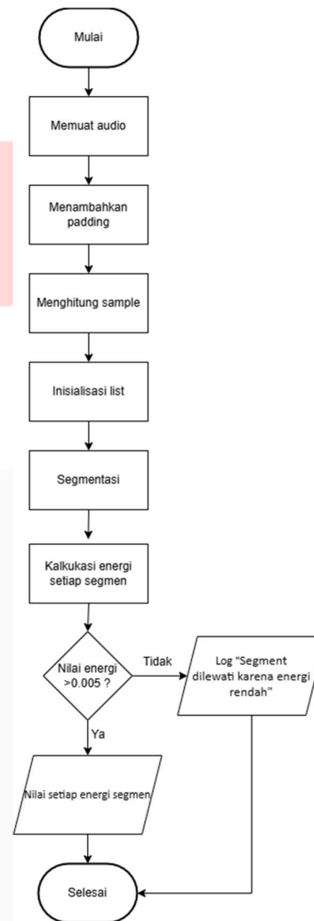
GAMBAR 1 Alur Segmentasi
