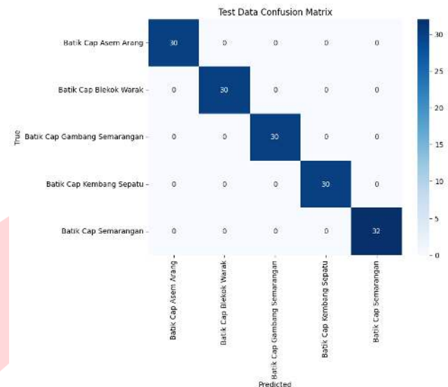
GAMBAR 8 (CONFUSION MATRIX)
