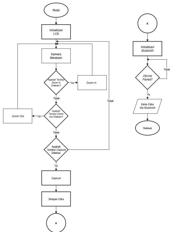
GAMBAR 3. Flowchart Algoritma Pemrograman
