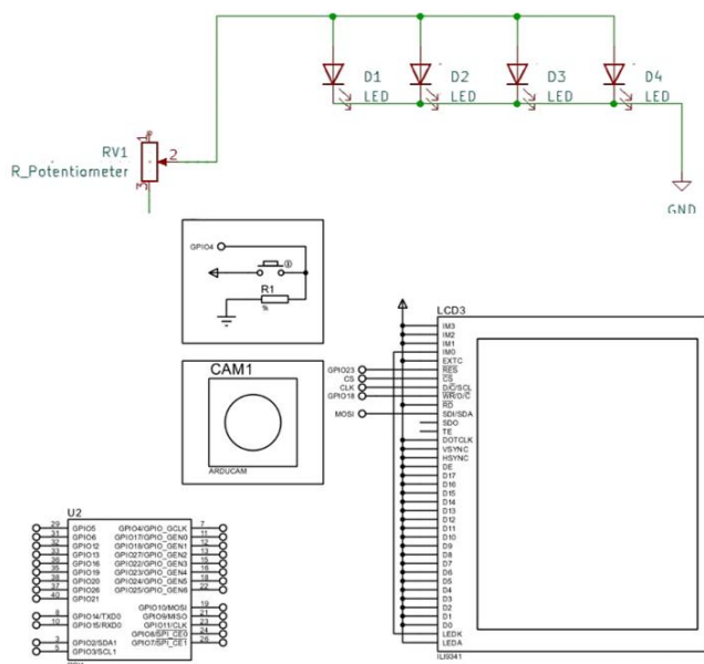
GAMBAR 2. Skematik Diagram Sistem
