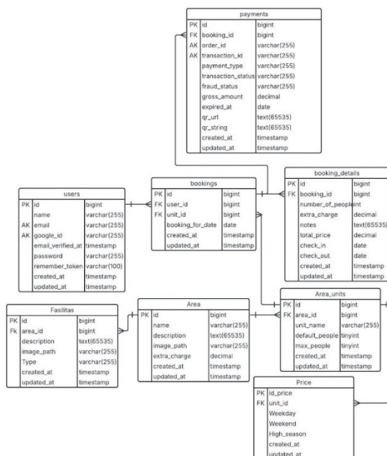
GAMBAR 3 Skema Database
