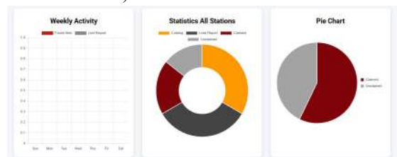
GAMBAR 10 Modul Statistik
