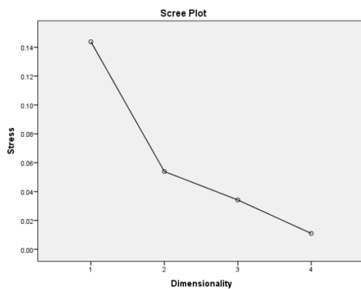
GAMBAR 4 Scree Plot Penentuan Jumlah Dimensi
