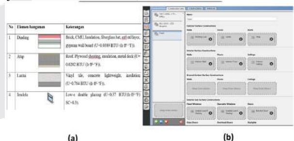
GAMBAR 3 (a) Nilai U material bangunan (b) Input pada simulasi.
