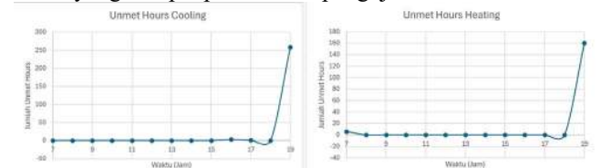
GAMBAR 11 Jumlah Unmet Hours Skema 2.
