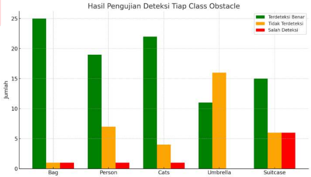
GAMBAR 4 Grafik evaluasi dari hasil pengujian posisi tetap dengan faktor tambahan
