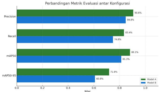
GAMBAR 2 Grafik perbandingan antar model
