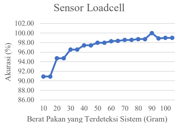
Gambar 13. Hasil Pengujian Keakuratan Sensor Loadcell
