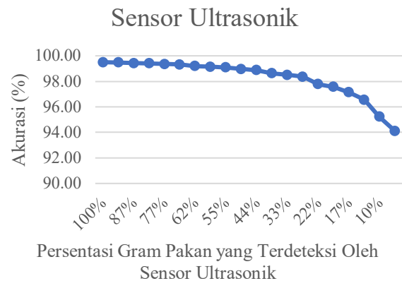
Gambar 12. Hasil Pengujian Keakuratan Sensor Ultrasonik
