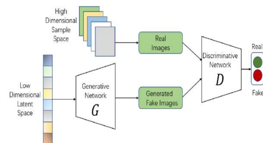
GAMBAR 5 Arsitektur VGAN
