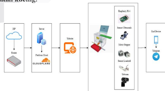
GAMBAR 1. DESAIN SISTEM
