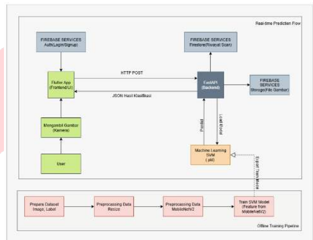
GAMBAR 1 Diagram Arsitektur Toxmap
