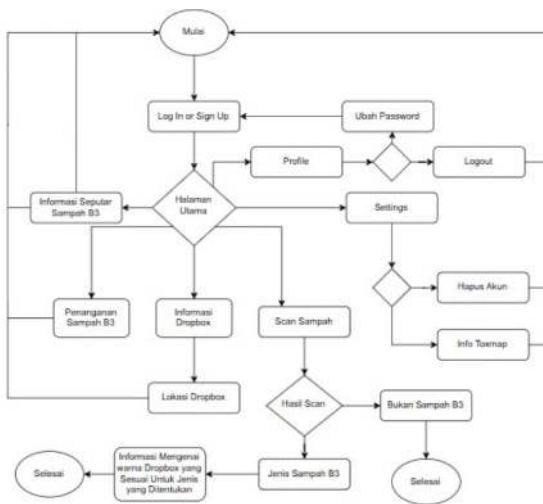
GAMBAR 2 Flowchart Navigasi Aplikasi Toxmap
