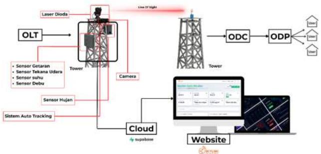
GAMBAR 8 Blok Diagram Sistem Keseluruhan
