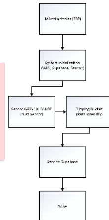
GAMBAR 1 Blok Sistem IoT
