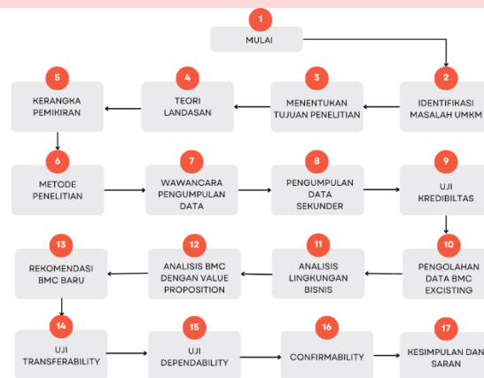
Gambar 3. 1 Tahapan Penelitian
