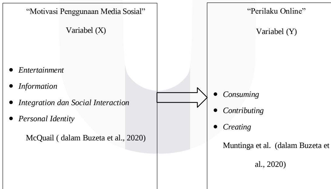
Gambar 2. 1 Kerangka Pemikiran
