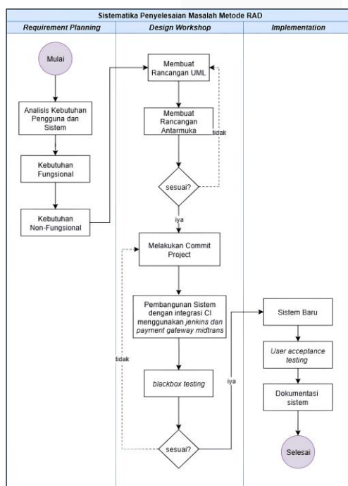
Gambar 3.1 Sistematika Metode Penyelesaian
