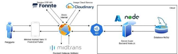
Gambar 1 (Arsitektur sistem RFC Store)
