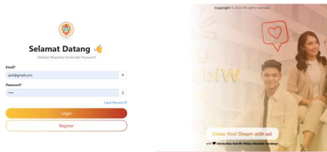
GAMBAR 11 Login Camaba
