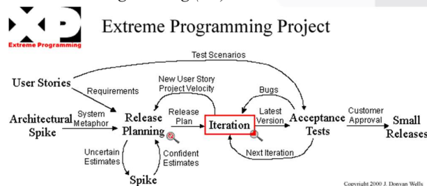
GAMBAR 1 Siklus XP Sumber: ExtremeProgramming.org
