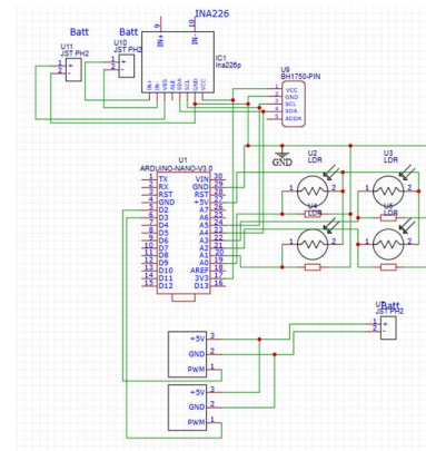
GAMBAR. 5 SKEMATIK
