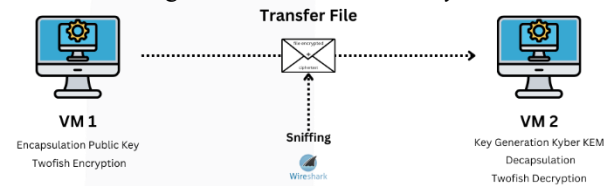
Gambar 7. Simulasi Virtual Machine (VM)
