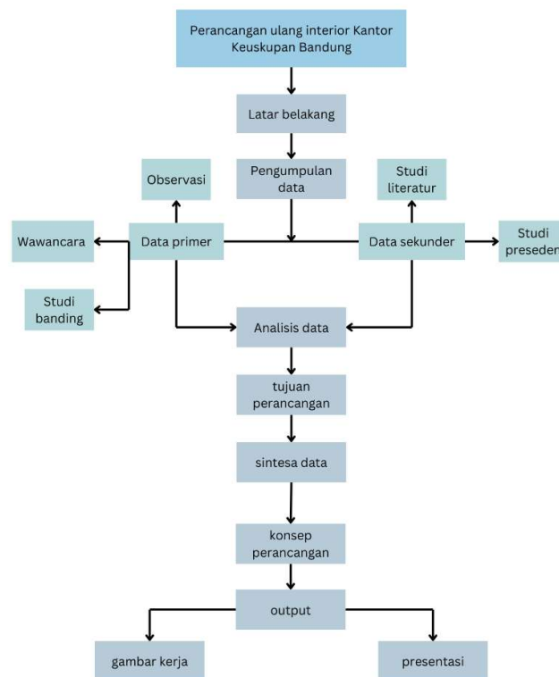
Gambar 1. 2 Kerangka Berpikir
