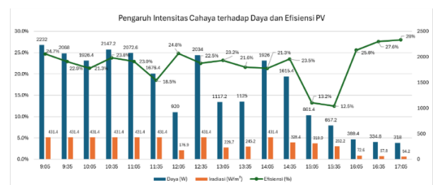
Gambar 6 Grafik Pengaruh Intensitas cahaya, Daya, dan Efisiensi Panel Surya
