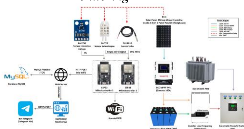
Gambar 1 Arsitektur Sistem Monitoring
