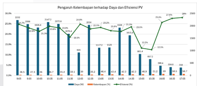
Gambar 8 Pengaruh Kelembapan lingkungan terhadap Daya dan Efisiensi
