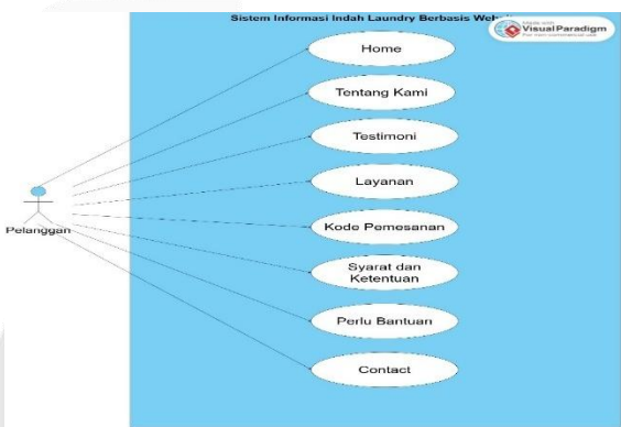
Gambar 1 Usecase Diagram pelanggan
