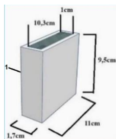
Gambar 3. 1 Desain Wadah
