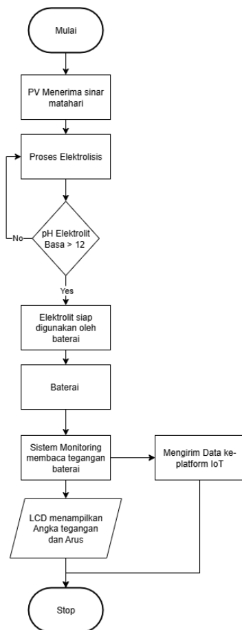
Gambar 3. 3 Diagram Alir
