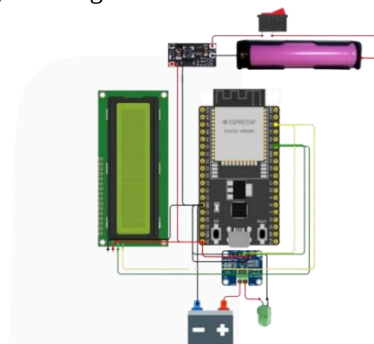
Gambar 3. 2 Diagram Pengkabelan
