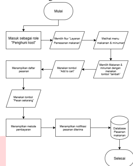
GAMBAR 2 Flowchart Fitur Penghuni Kost
