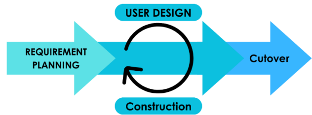
Gambar II-1 Metode RAD
