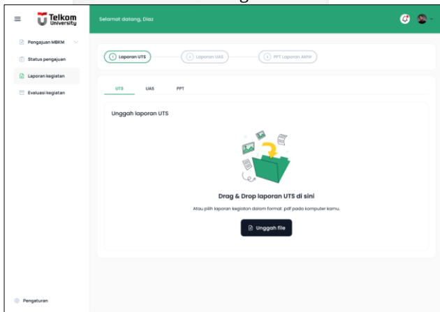
Gambar IV-6 Tampilan Menu
