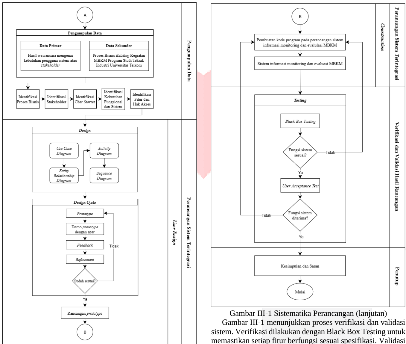
Gambar III-1 Sistematika Perancangan (lanjutan)
