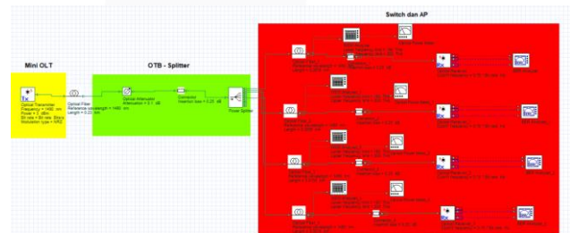
Gambar 5 Simulasi Optisystem
