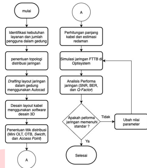
Gambar 1 Diagram alur perancangan jaringan
