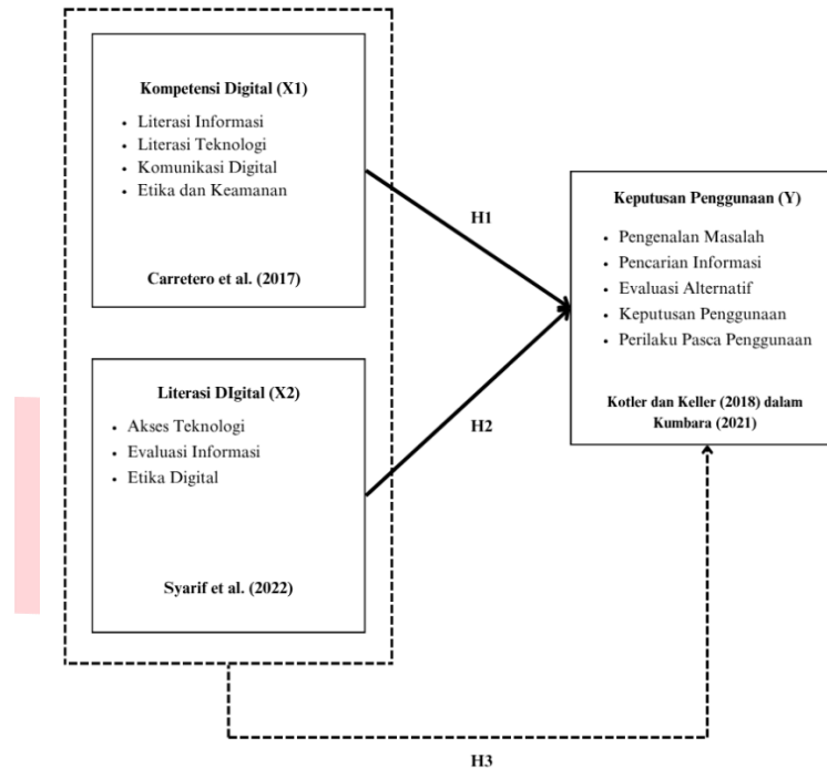
Gambar 2. 1 Kerangka Pemikiran
